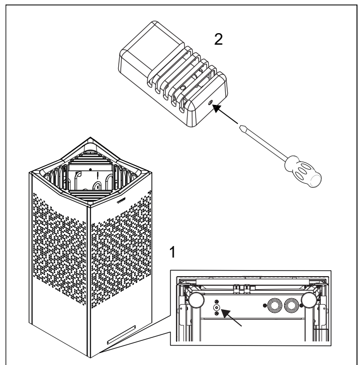
Abbildung 2: Zurücksetzen des Überhitzungsschutzes
