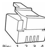
Steckerbelegung eines RJ10-Anschlusses
