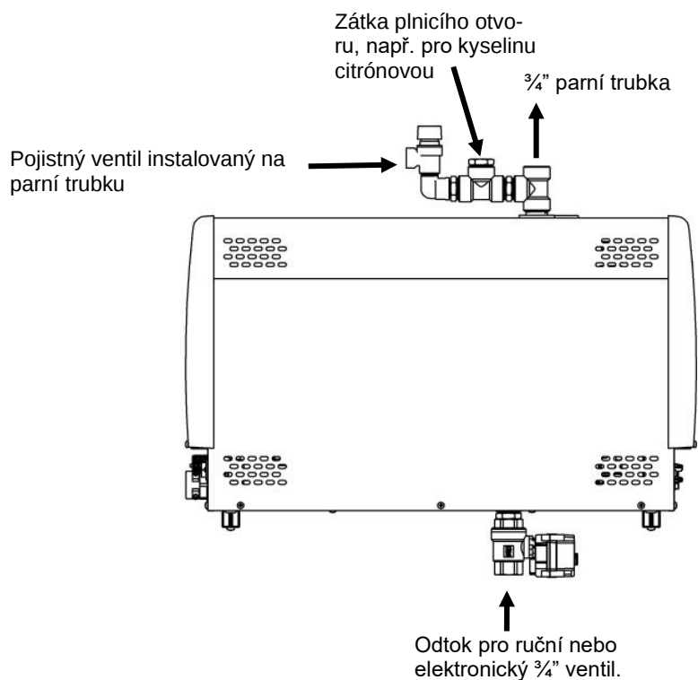
Obrázek. Instalace pojistného ventilu a automatického vypouštěcího ventilu (Příslušenství automatic drain valve). Viz schéma obvodu zapojení.
