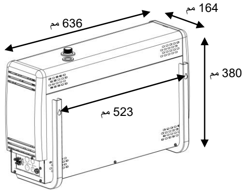
تركيب مولد البخار بالحائط
