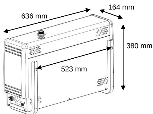
Support mural du générateur de vapeur
