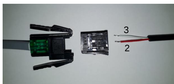
Připojení kabelu snímače teploty
