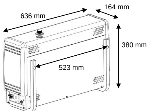
Montáž generátoru páry na stěnu
