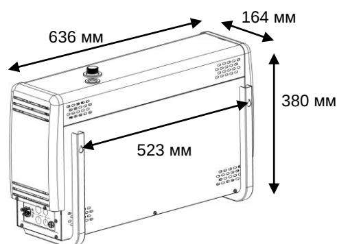
Настенный монтаж парогенератора
