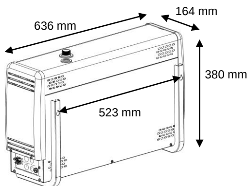
Montaggio a parete del generatore di vapore
