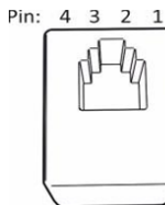
Penindeling van een RJ10-printplaatstekker
