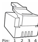
Rozvržení pinů konektoru RJ10
