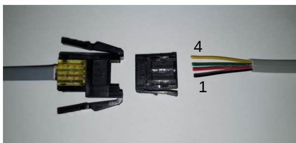
Připojení kabelu ovládacího panelu
