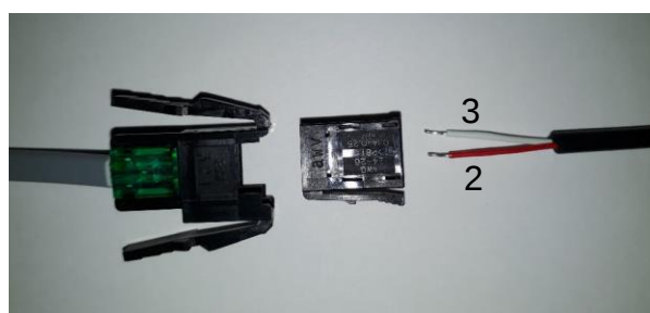
Anslutning av temperatursensorns kabel
