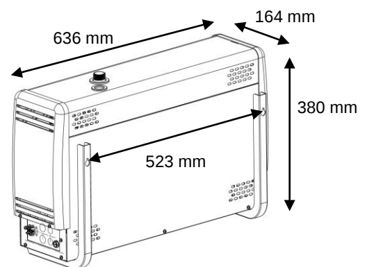
Wandmontage des Dampferzeugers
