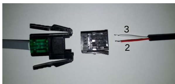
Lämpötila sensori kaapelien kytkentä
