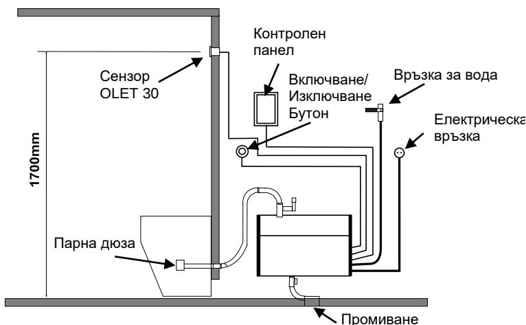
Монтаж на контролния панел
