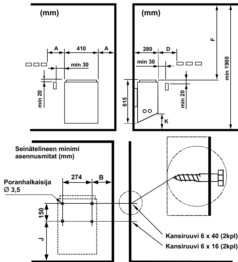
Kuva 2. Suojaetäisyydet
