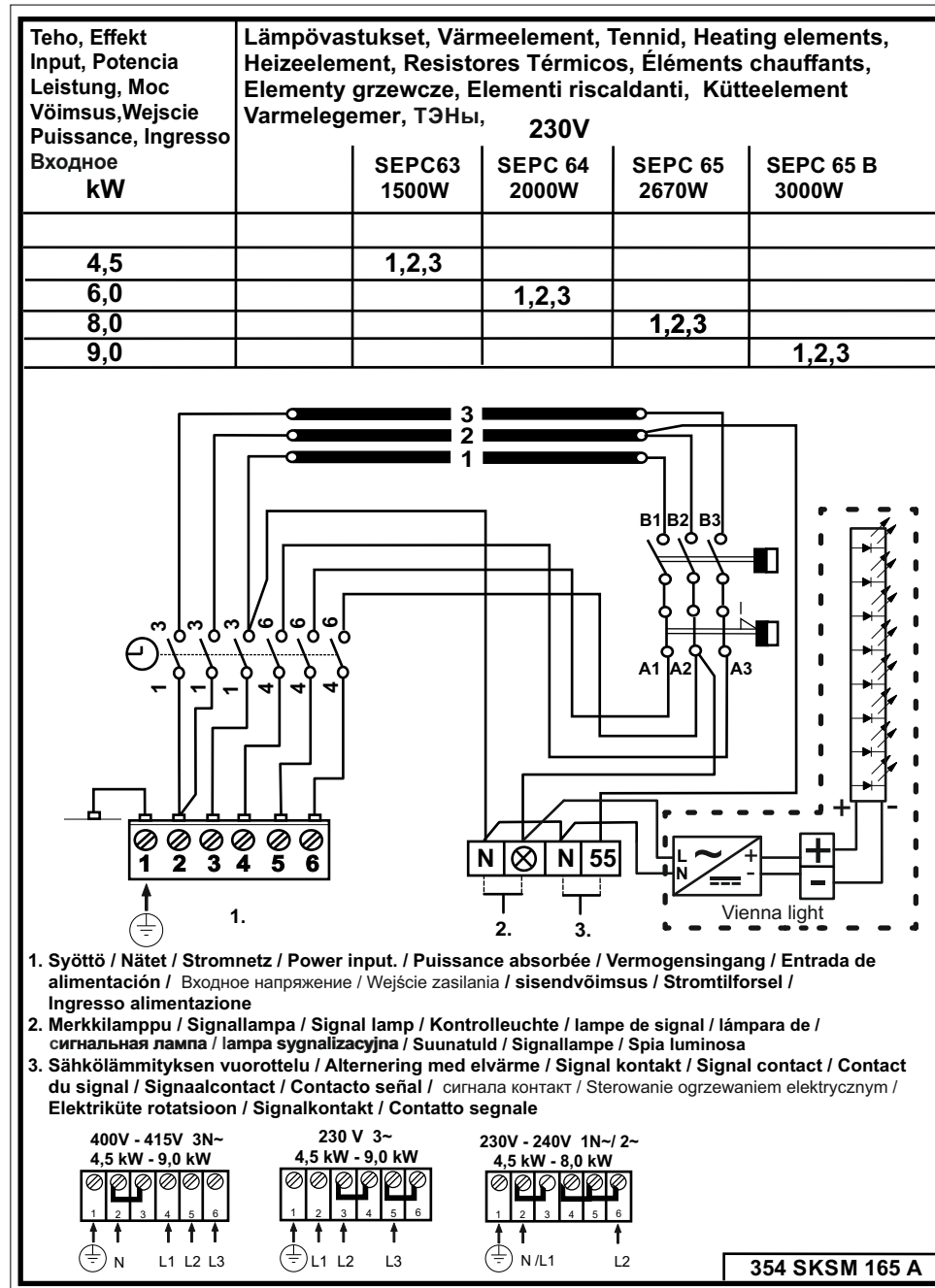
Abbildung 4. Schaltdiagramm
