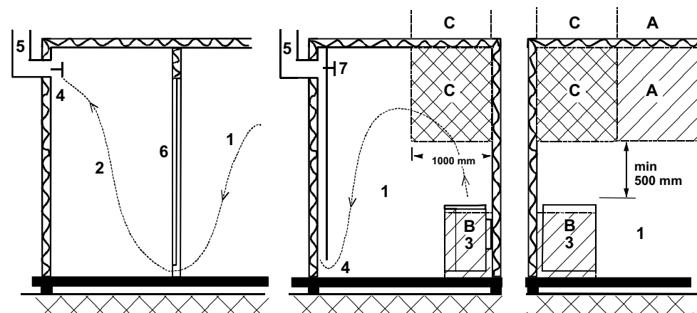
Kuva 1. Suositeltava ilmanvaihto saunassa
