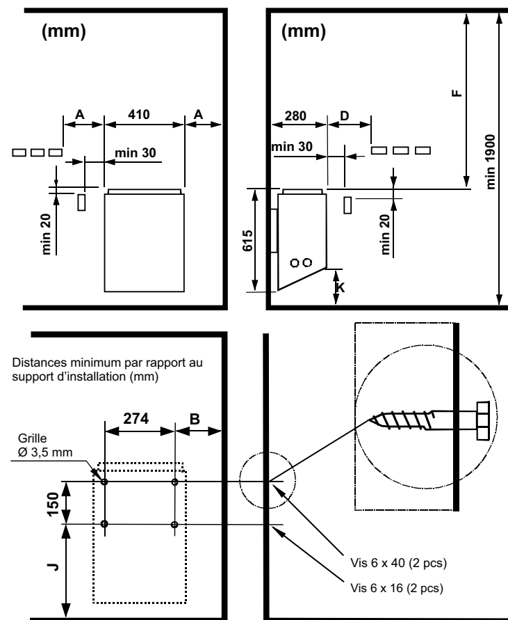
Illustration 2. Dégagements de sécurité
