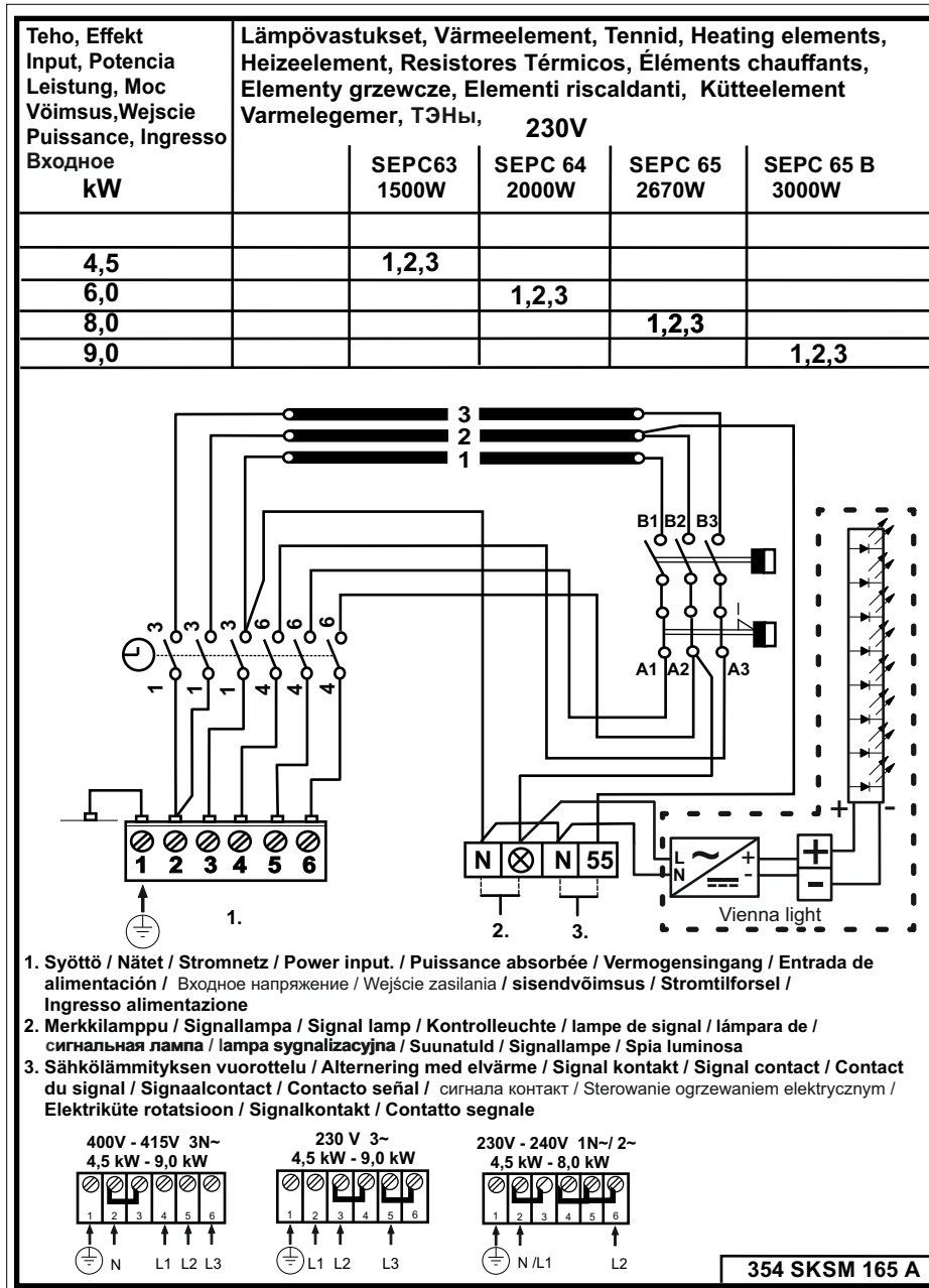
Kuva 4. Kytentäkaava
