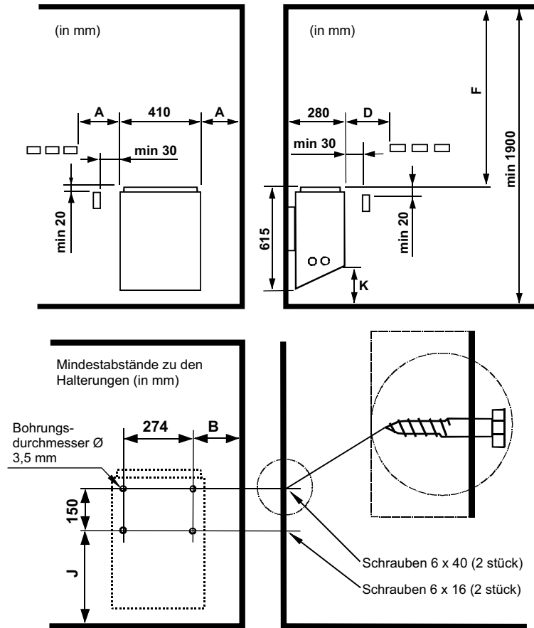
Abbildung 2. Sicherheitsabstände
