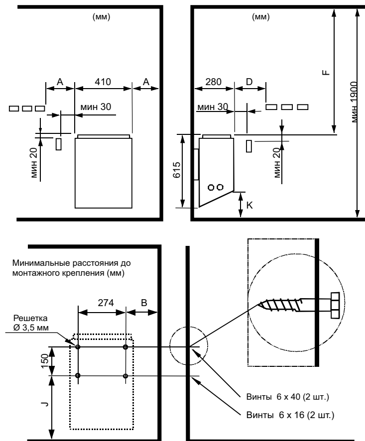
Рис. 2 Безопасные расстояния
