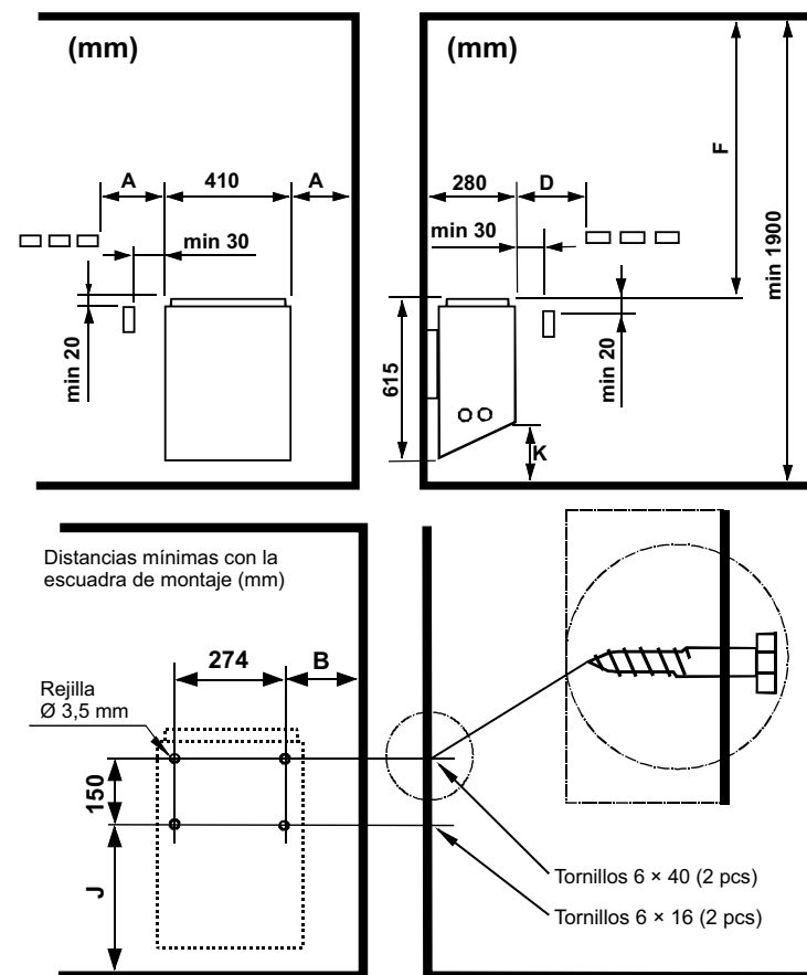
Imagen 2. Separación de seguridad
