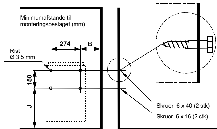
Billede 2. Sikkerhedsafstande
