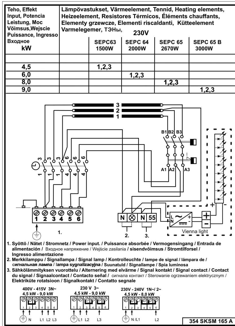
Rysunek 4. Schemat podłączenia pieca
