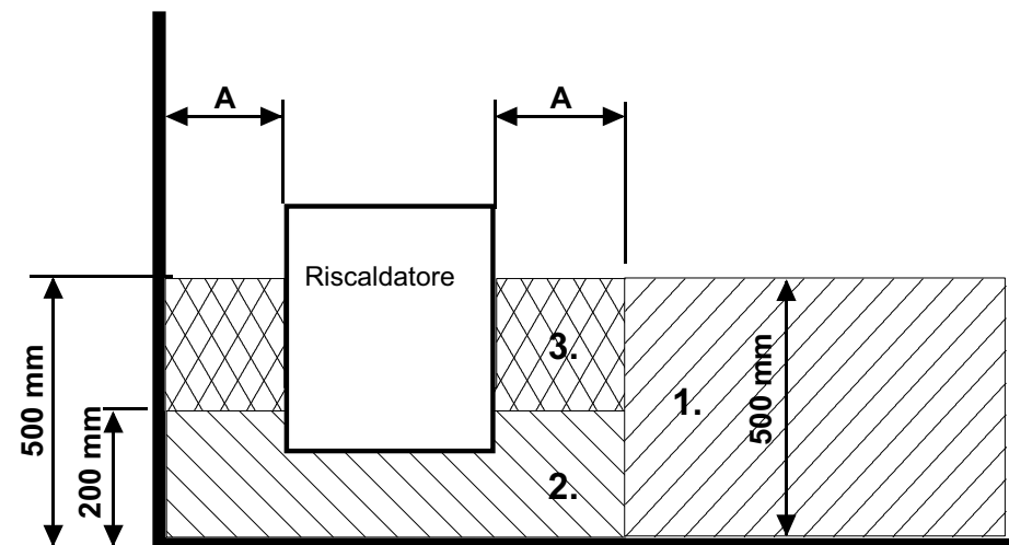
Immagine 3. Collocazione della scatola dei collegamenti
