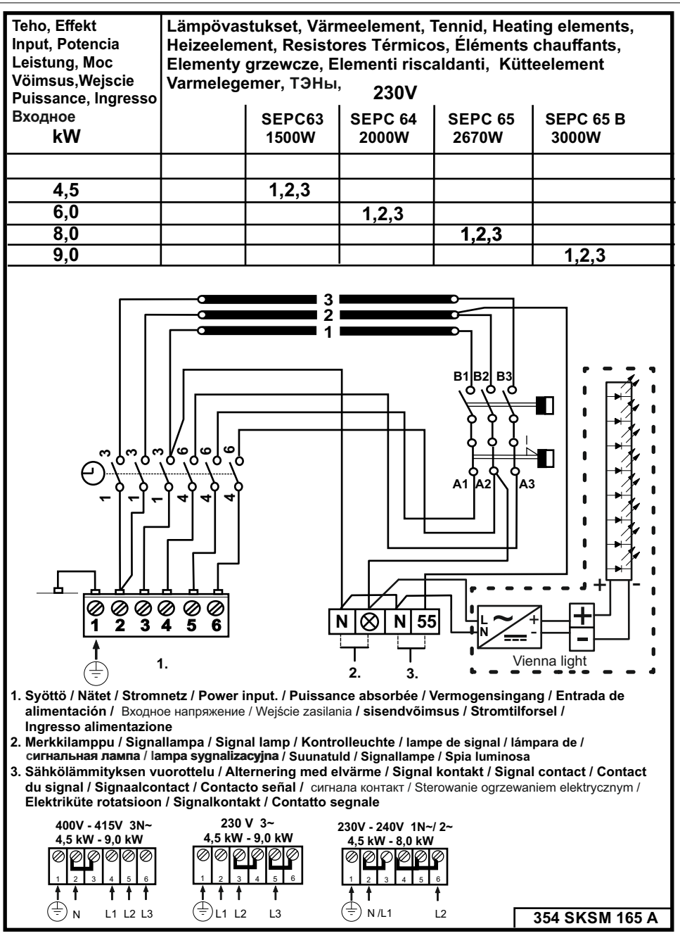
Immagine 4. Diagramma dei collegamenti
