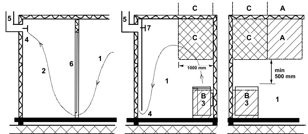
Imagen 1. Ventilación recomendada para la sauna.
