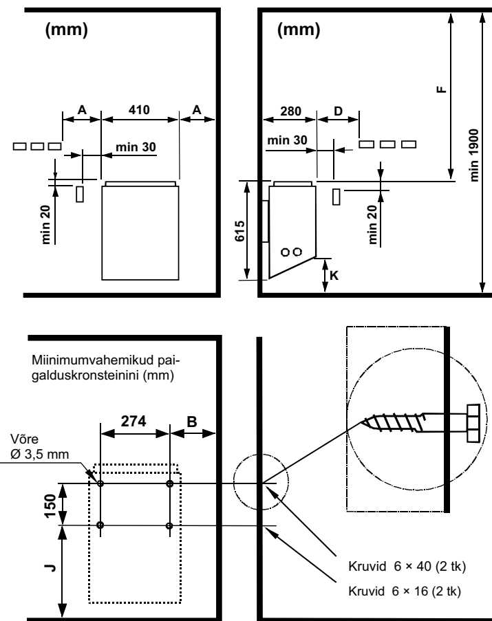
Joonis 2. Ohutusvahemikud
