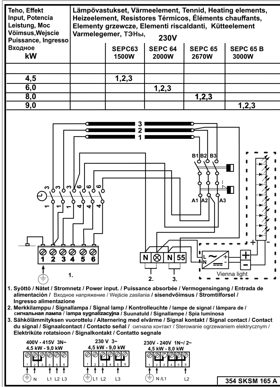
Bild 4. Kopplingsschema
