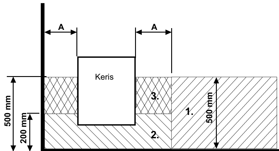
Joonis 3. Lavaruumis ühenduskaabli ühenduskarbile sobiva koha leidmine
