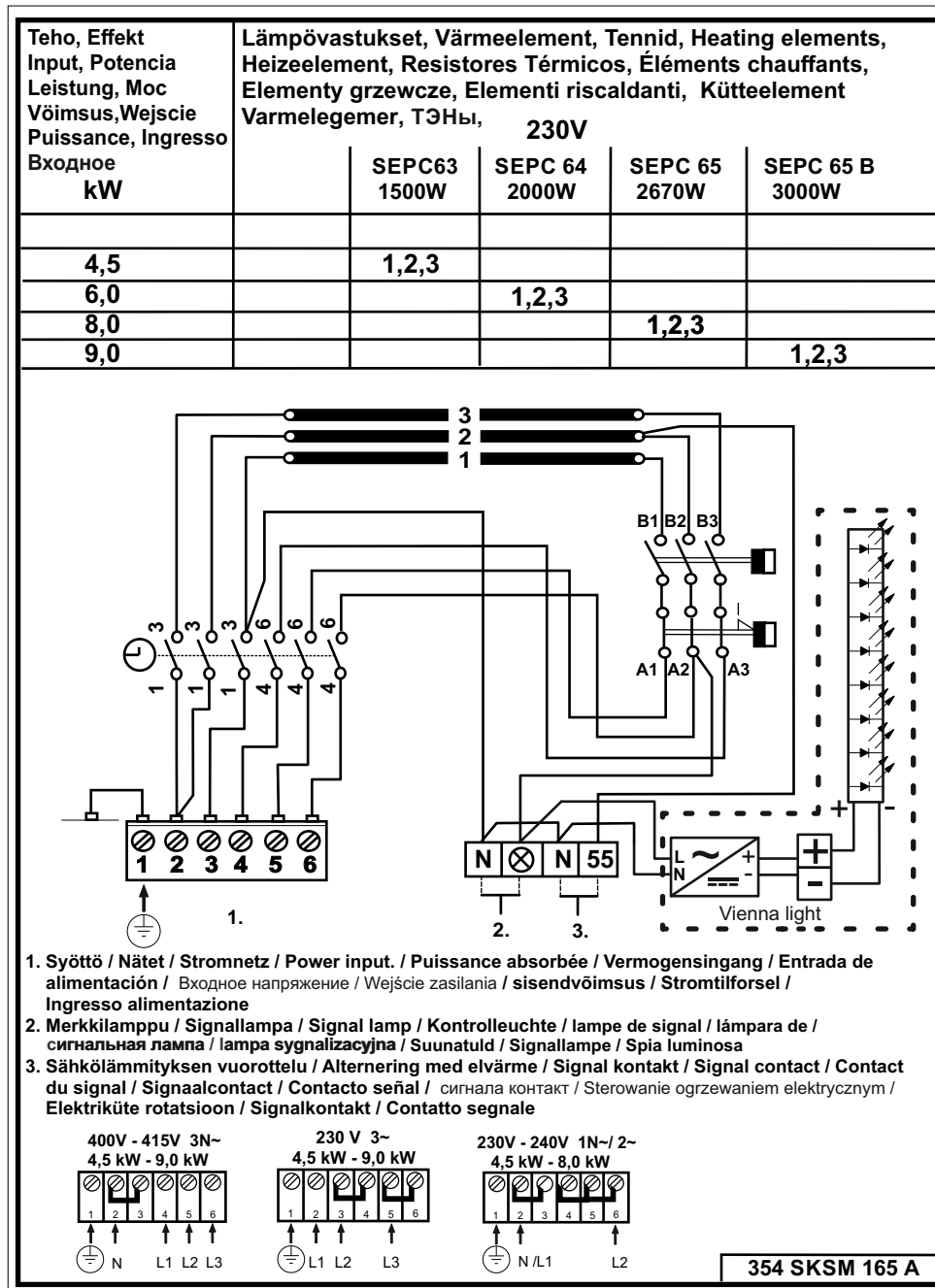
Illustration 4. Schéma de raccordement
