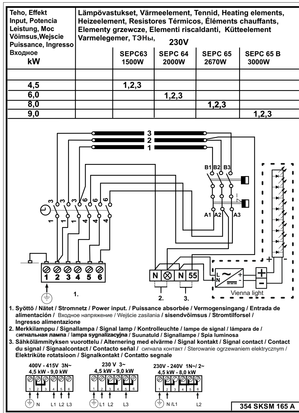
Imagen 4. Diagrama de conexiones
