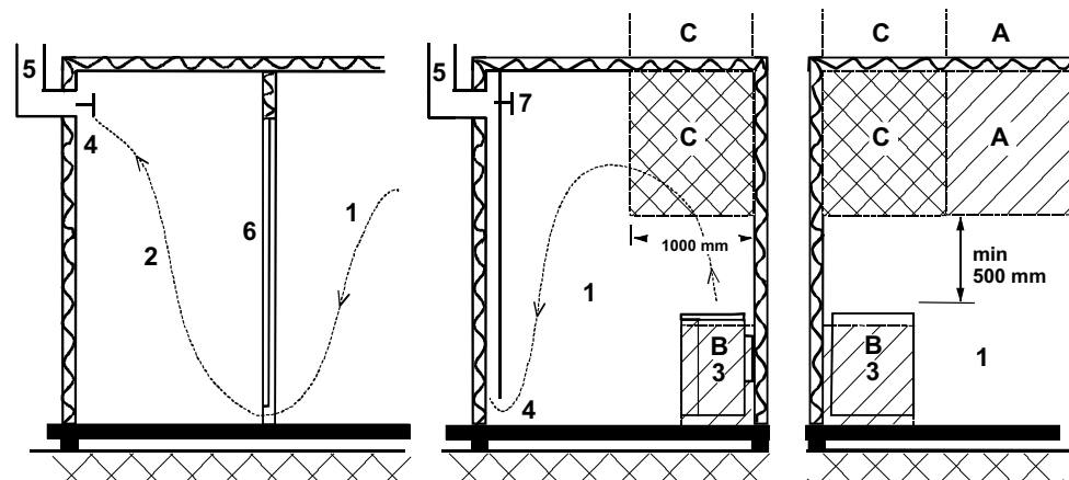
Bild 1. Rekommenderad ventilation i bastun
