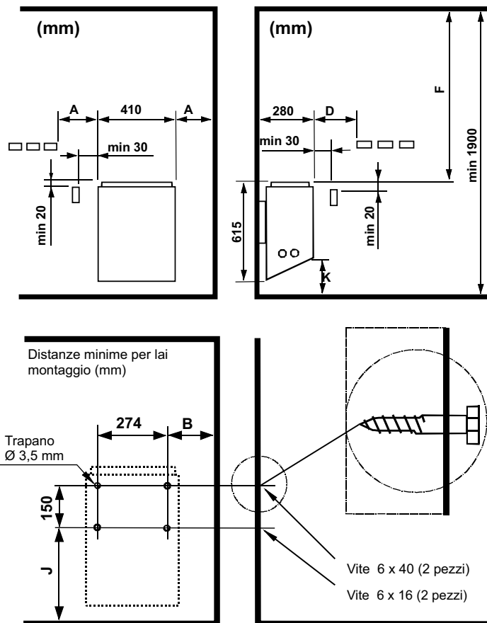
Immagine 2. Distanze di sicurezza del riscaldatore e posizione del sensore alla parete
