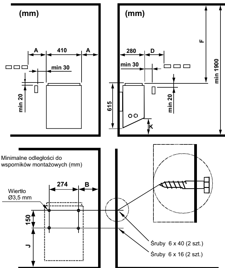
Rysunek 2. Bezpieczne odległości
