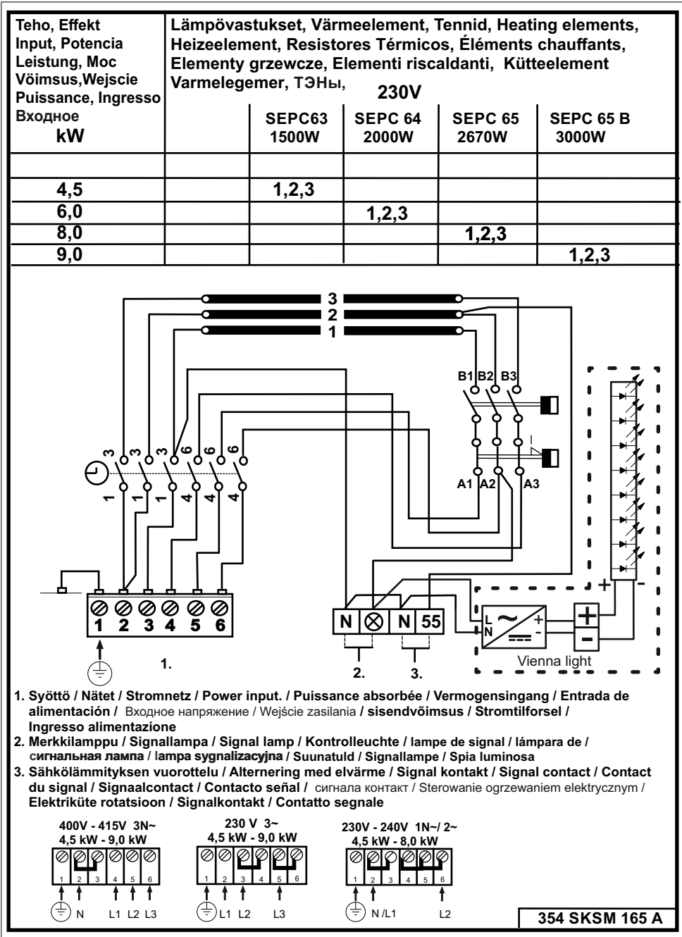
Billede 4 Ledningsdiagram
