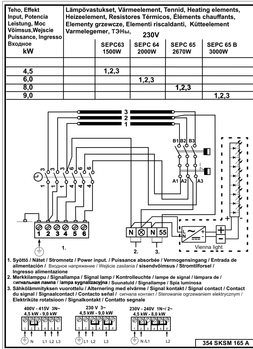
Рис. 4 Схема электрических соединений
