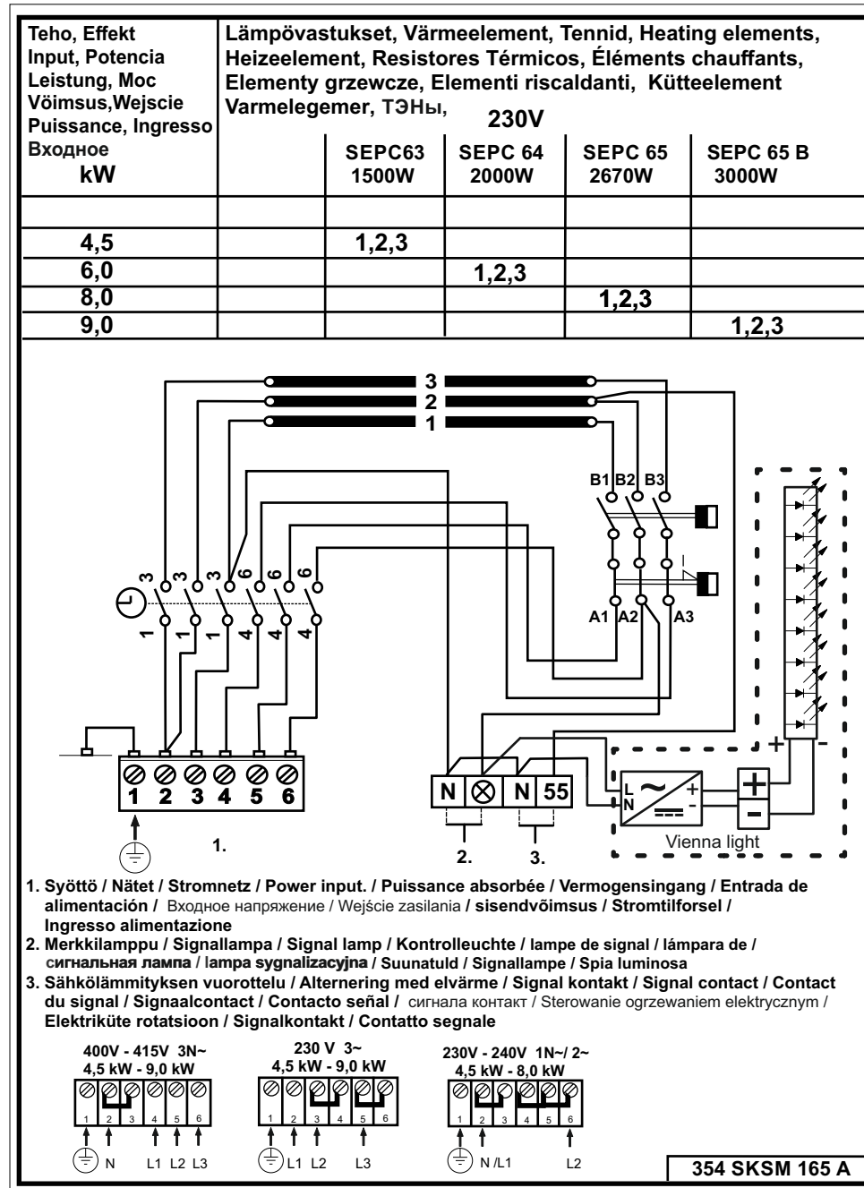
Joonis 4. Ühenduste skeem
