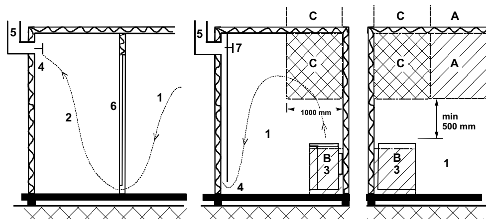
Abbildung 1. Empfohlene Belüftung des Saunaraums
