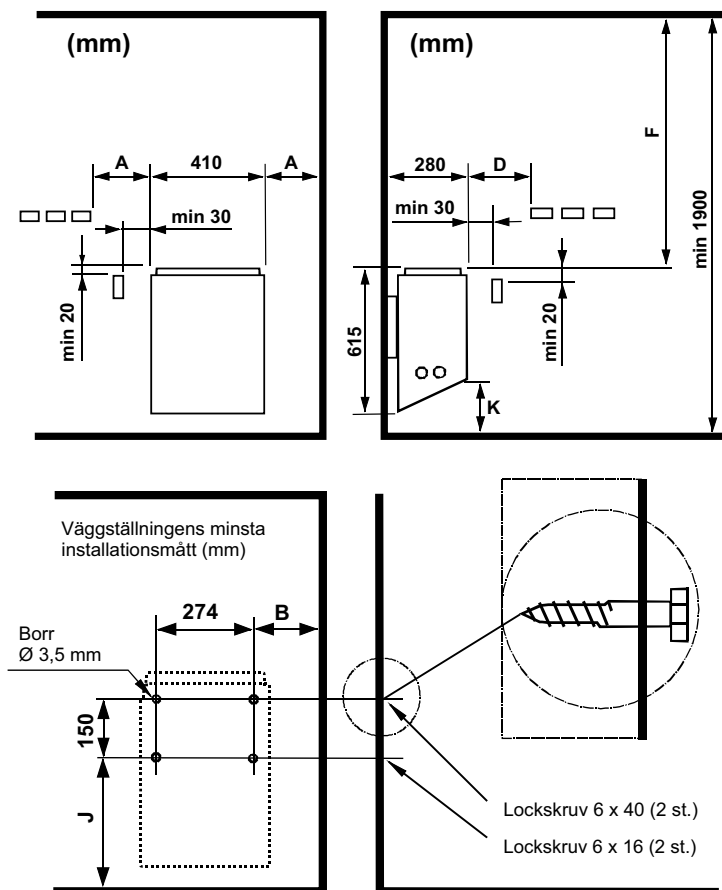
Bild 2. Skyddsavstånd
