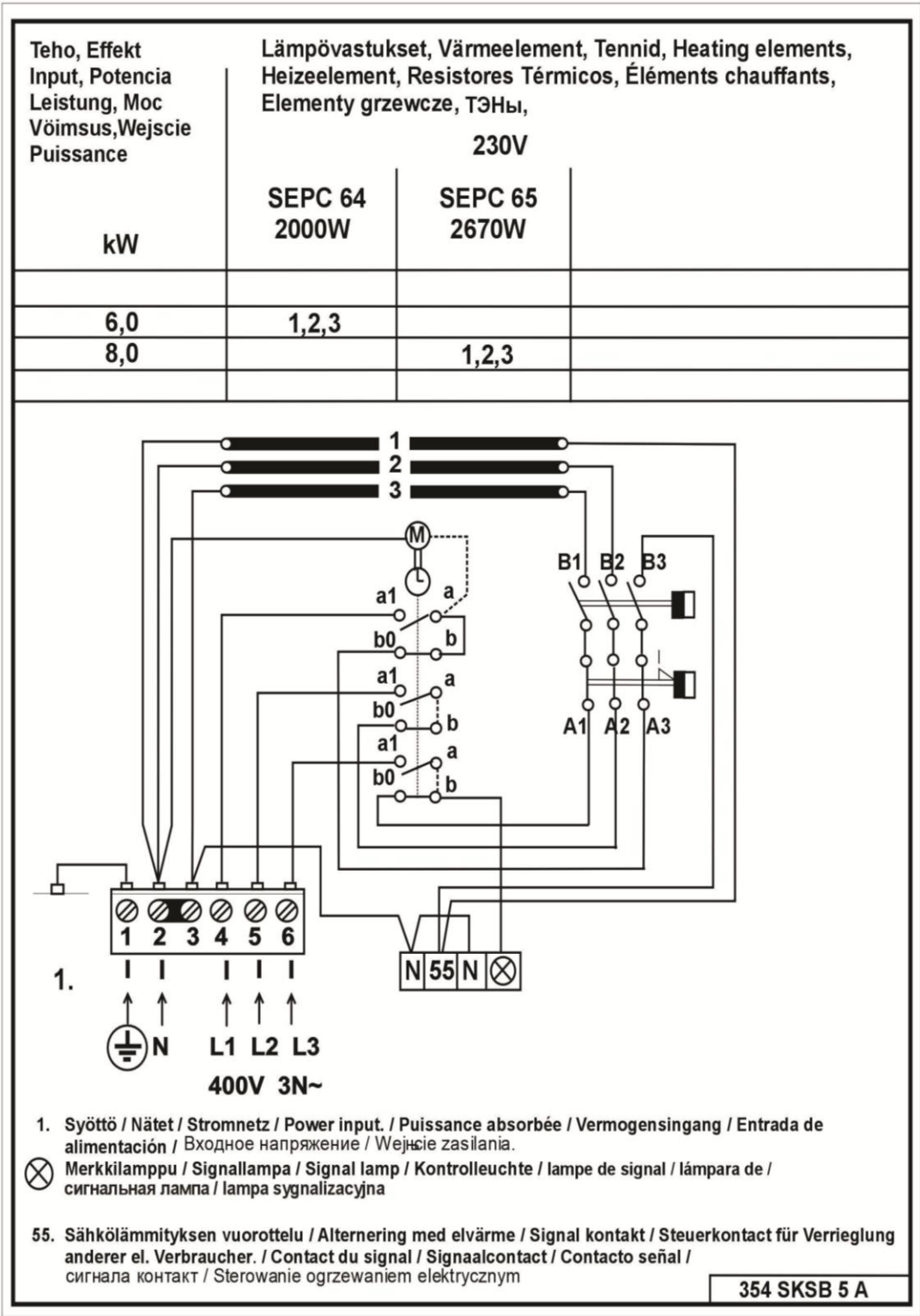
Illustration 4 Schéma de raccordement
